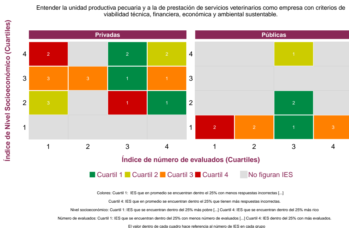
Figura 10: Mapa de calor. Relación del nivel socioeconómico, número de estudiantes evaluados y desempeño, por sector - Afirmación 5
