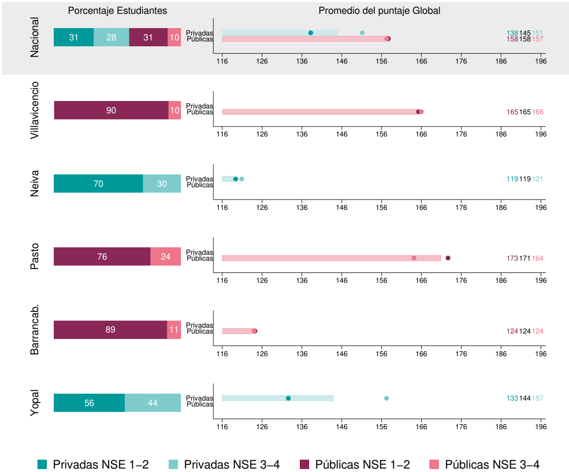
Figura 12: Puntaje promedio por sector y NSE para municipios representativos en la prueba Saber Pro 2017 - Continuación
